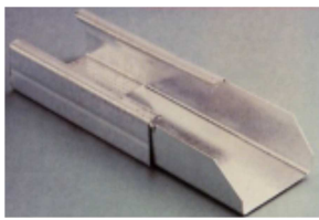
Giunzione 49*15/49*27
