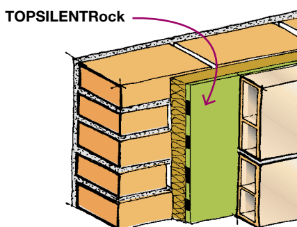
TOPSILENTRock versione non imbustata Faccia verde rivolta verso l'operatore in fase di montaggio
