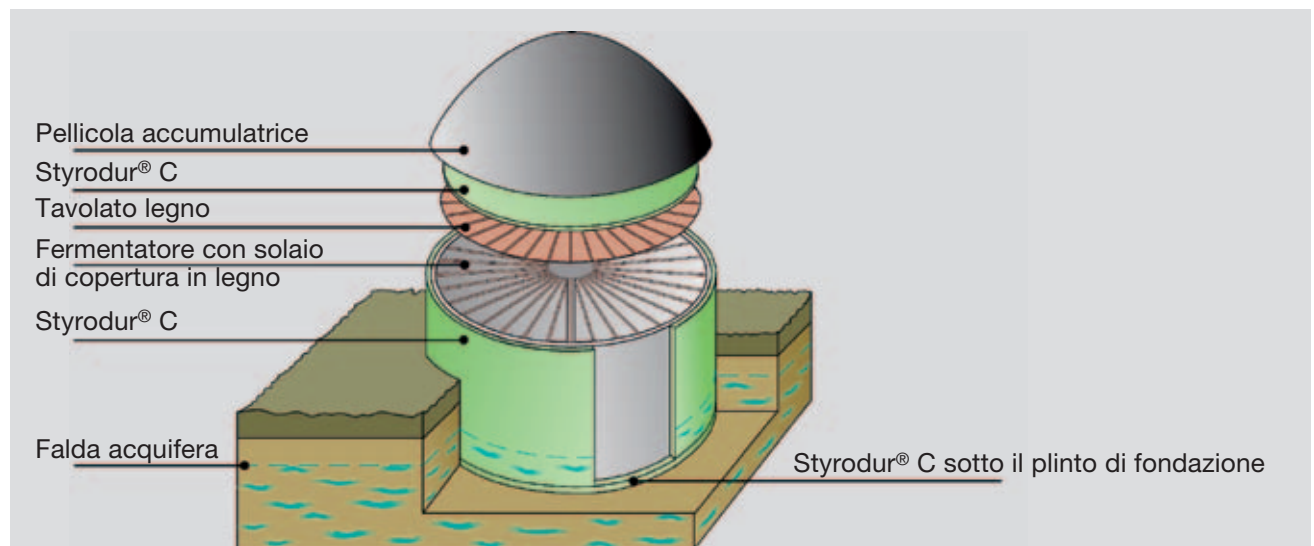
Fig. 2: Rappresentazione schematica di un fermentatore con copertura a pellicola.
