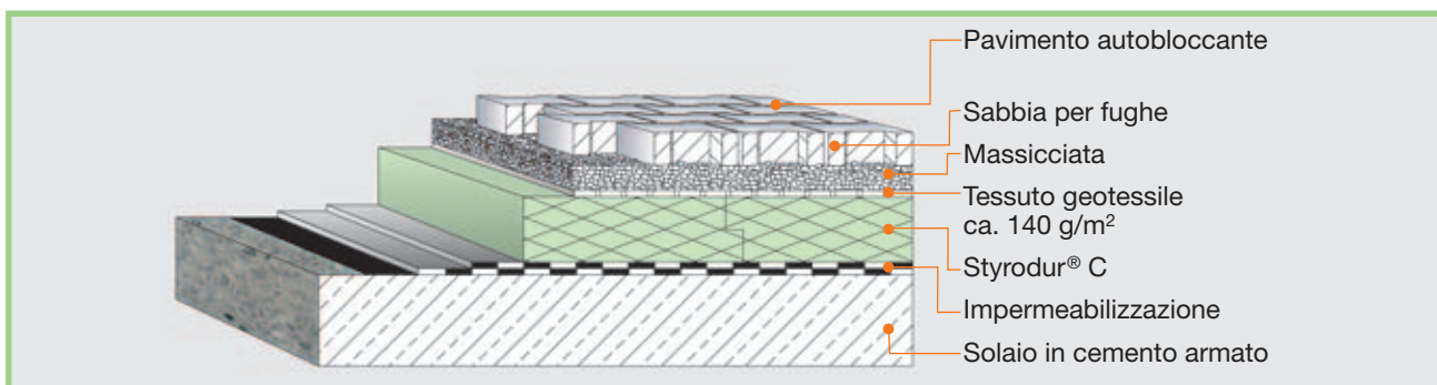
Fig. 4: Tetto rovescio con strato di protezione superficiale in ghiaia.
